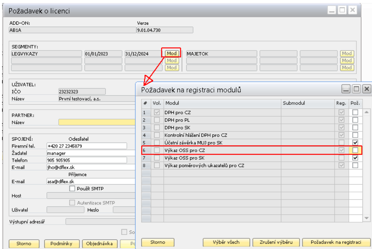
Obr. 1 Požadavek o licenci s registrací modulů
